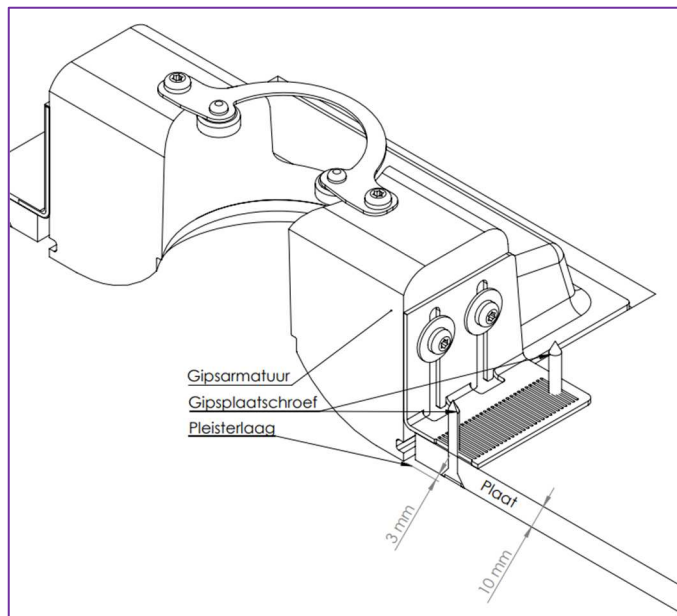
Fig. 5: Voorbeeld maatvoering voor de montage van het gipsarmatuur (let op! doorsnede)
