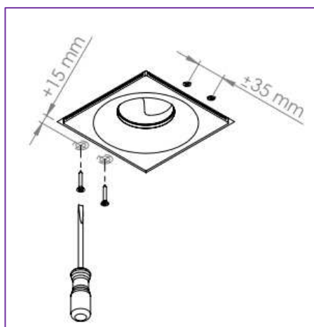
Fig. 4: Vast schroeven gipsarmatuur in het plafond
